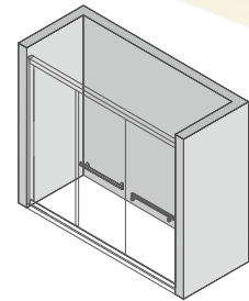
Model: 418-4 尺寸：宽度 1200mm-2400mm 高度 2000-2200mm 开门方式：双活动移门 + 一固定 形状：一字型平移门 边框：304 不锈钢镜光
