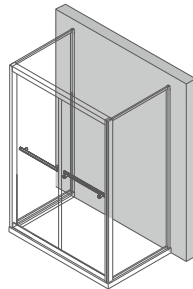
Model: 418-U 尺寸：宽度 1200mm-2200mm 高度 2000-2200mm 侧固 300mm-1000mm 开门方式：双活动移门 + 两转角 形状：U 形平移门 边框：304 不锈钢镜光
