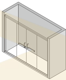
Model: 418-7 尺寸：宽度 1200mm-2400mm 高度 2000-2200mm 开门方式：两固两活移门 形状：一字型平移门 边框：304 不锈钢镜光
