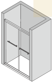
Model:418-5 Shower Room 淋浴房 订造范围：宽度 1100-2200MM 高度 1500-2200MM 开门方式：双活移门 石 基：80MM 宽 边 框：304 不锈钢 玻 璃：8MM 防爆玻璃
