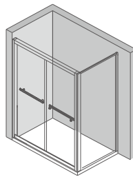
Model: 418-8 尺寸：宽度 1200mm-2200mm 高度 2000-2200mm 侧固 300mm-1000mm 开门方式：双活动移门 + 转角 形状：方形平移门 边框：304 不锈钢镜光
